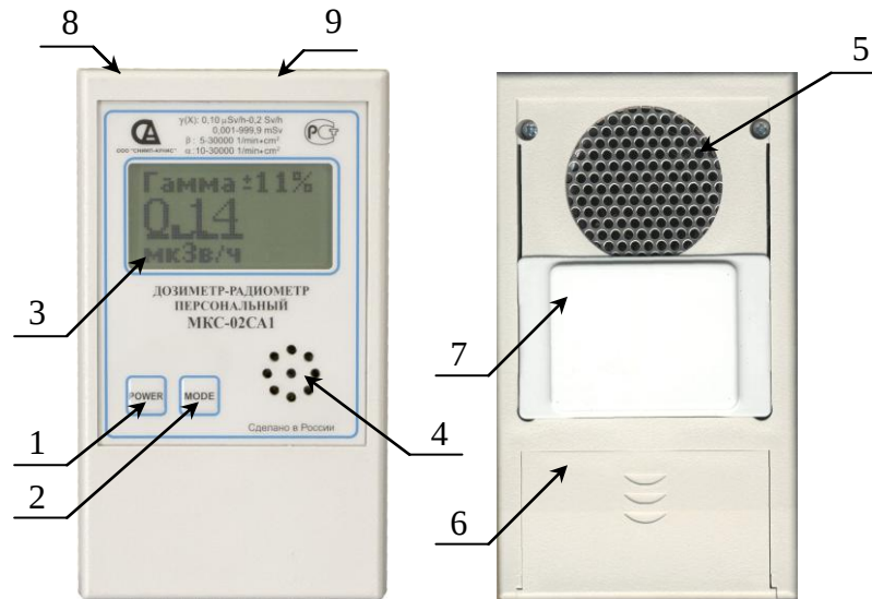
Рис. 1. Общий вид прибора MKC-02CA1
