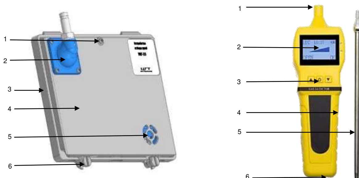
Рисунок 6.3 – Комплект отбора проб (газа/воздуха)
