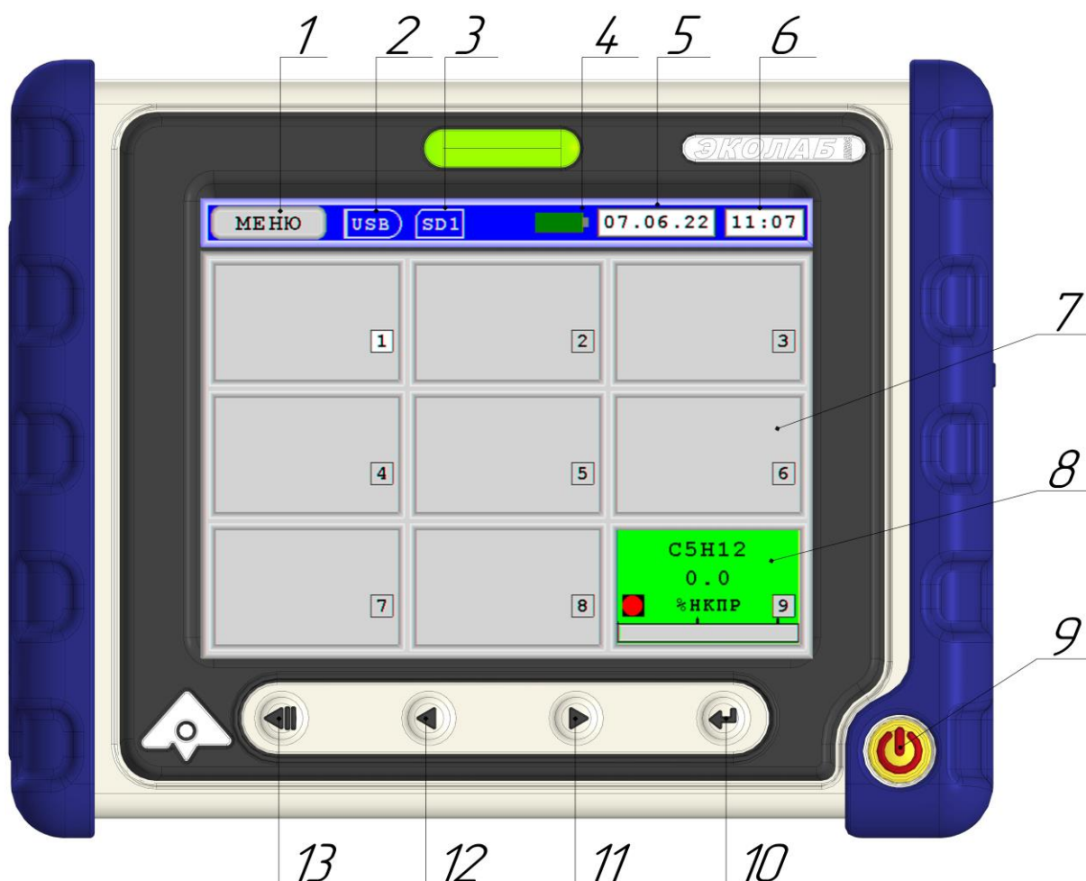
Рисунок 9.2 – Рабочий экран
