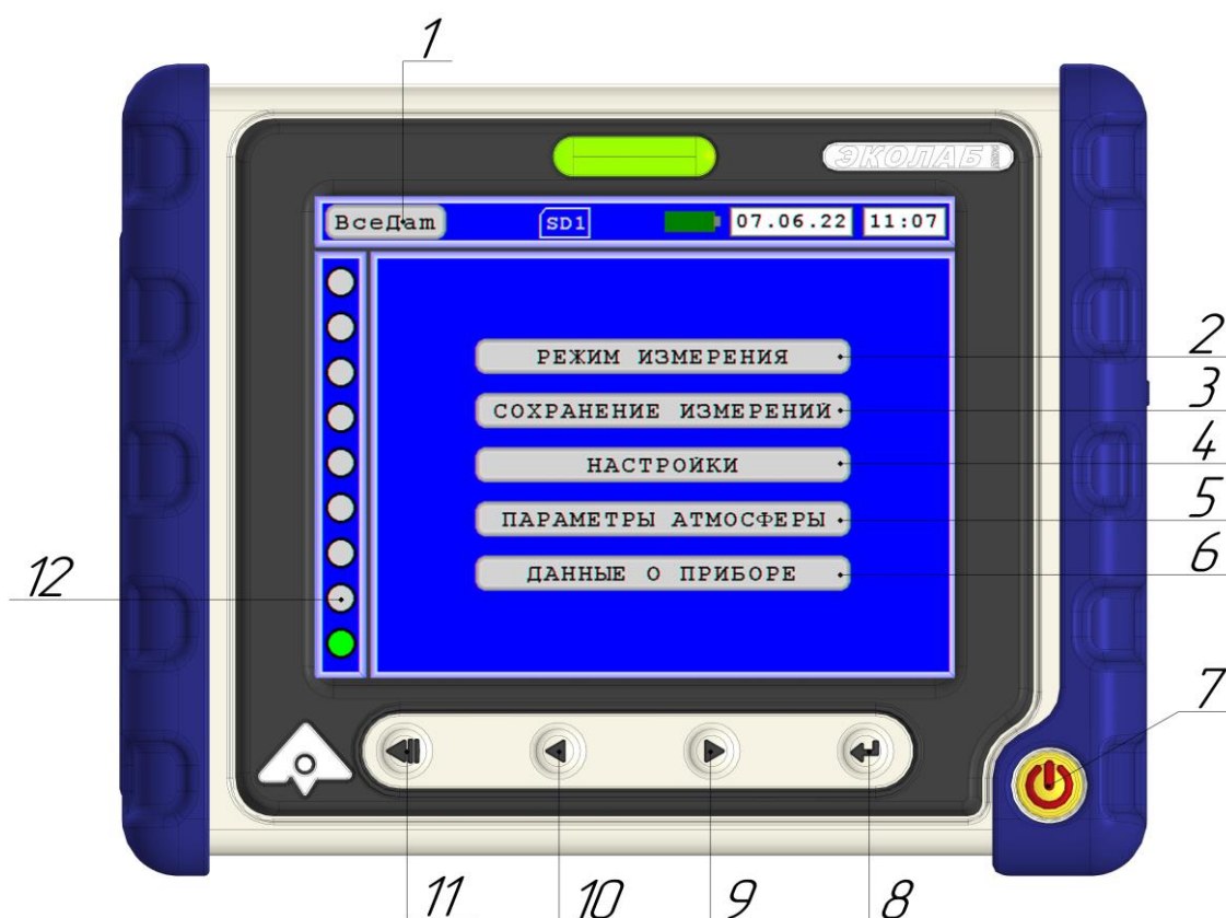
Рисунок 9.4 – Основное меню
