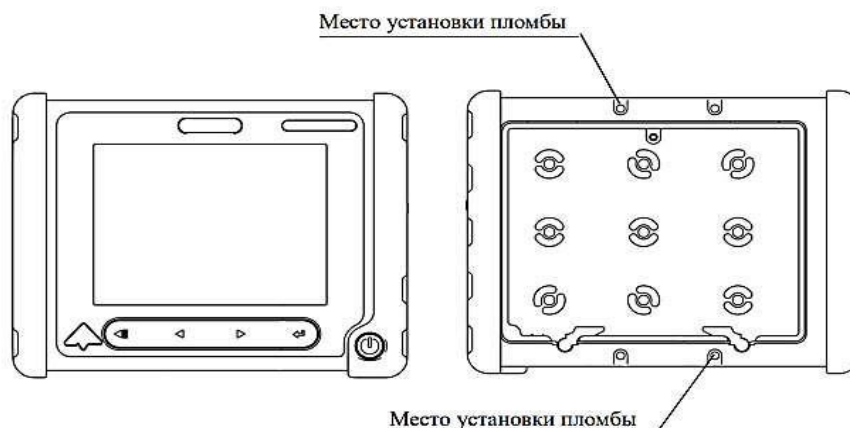
Рисунок 5.1 – Схема пломбировки
