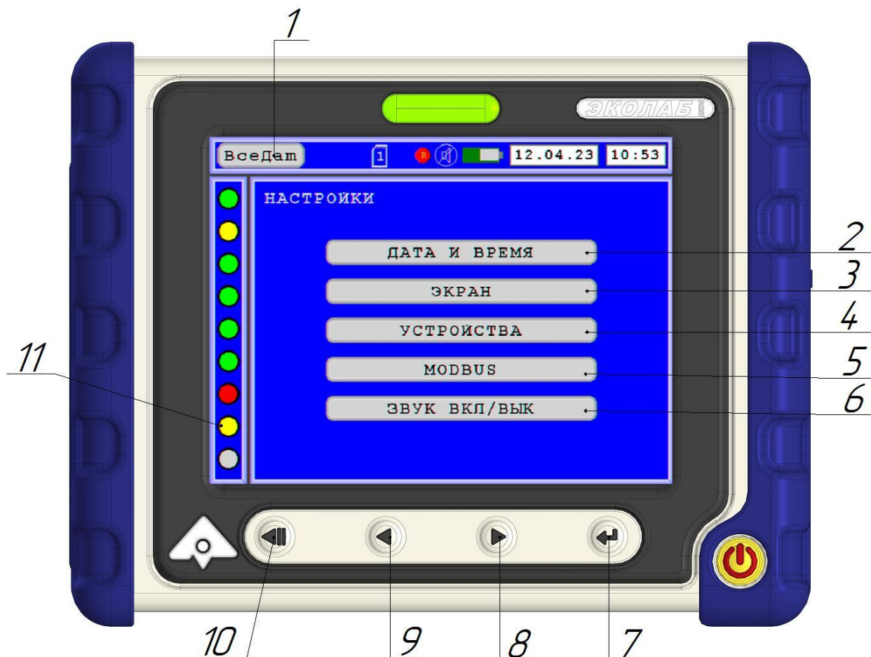
Рисунок 9.8 – Экран «НАСТРОЙКИ»
