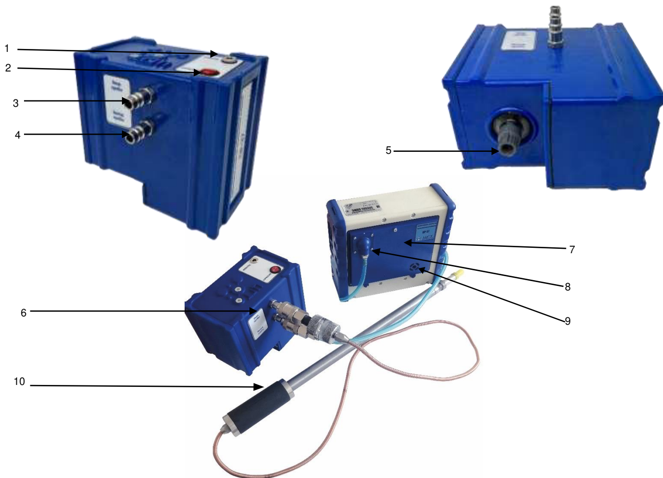
Рисунок 6.4 – Общий вид ПР-37
